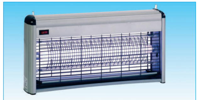
850020. Insecticida eléctrico de 15 W. con 1 lámpara de 15 W. Tamaño : Ancho : 50 cm. Alto : 26 cm. Fondo : 8 cm.
