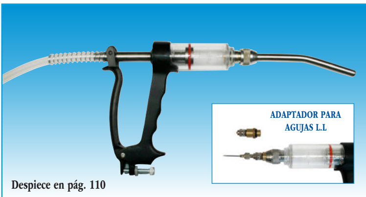
200910. DOSIFICADOR MP - 30 ml. Mango metálico y cilindro de plástico transparente. Graduado de 5 ml hasta 30 ml. ( Sin mochila ).
