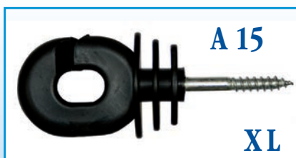
Anillo ext. Ø : 40 mm Gota de agua : 22 mm Tirafondo long. : 40 mm
